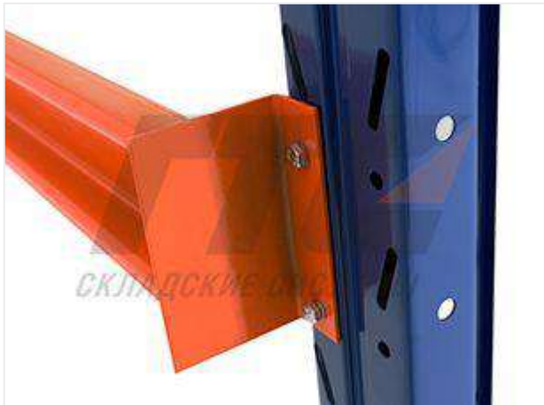
31 Ограничитель крепится на два Болта M8x35 с каждой стороны.
